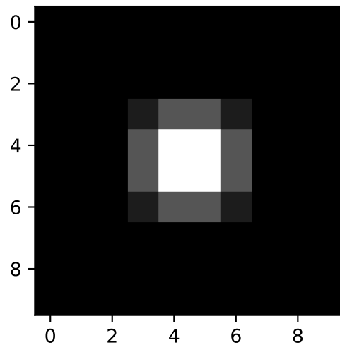
Linear (10, 10)
